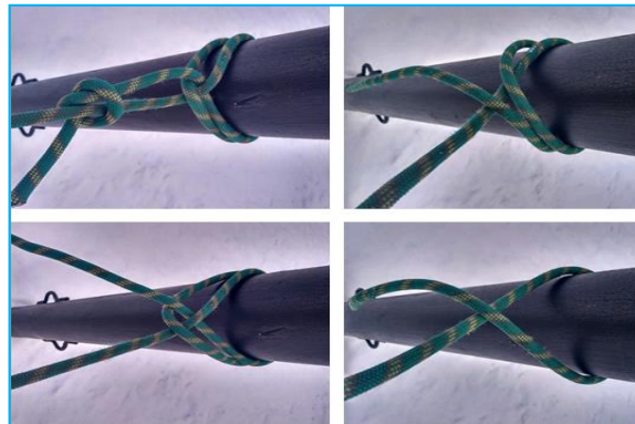
Узел стремя на опоре
